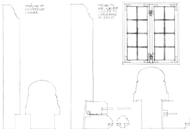
Nye vinduer med oprindelig profilering af poste og karme. Tegning: Steffen M. Søndergaard.
