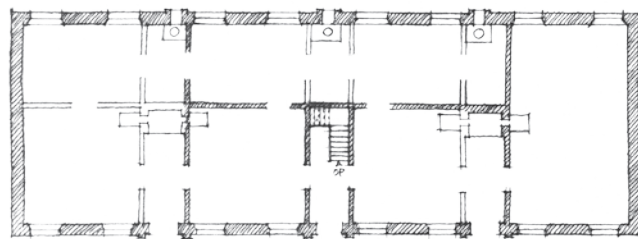
Rekonstruktion af hovedfacade og plandisposition. Skravering markerer registrerede forhold. Skitser: Steffen M. Søndergaard.
