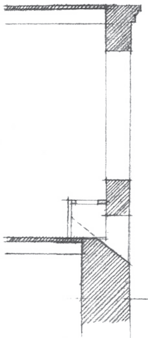
Nørre Vosborgs vestlænge med spor efter lokumsafløb samt principskitse. Foto og principskitse: Steffen M. Søndergaard.
